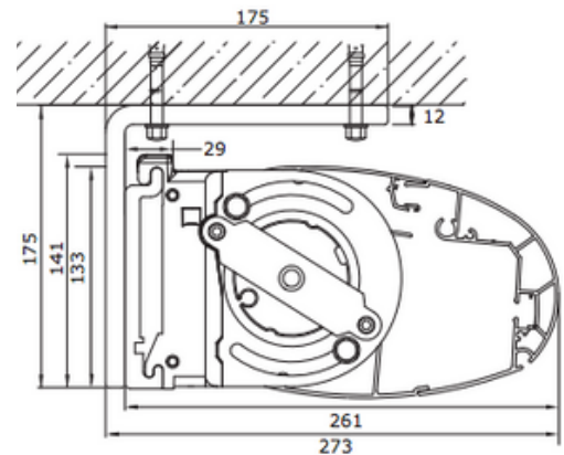
Plafondmontage
