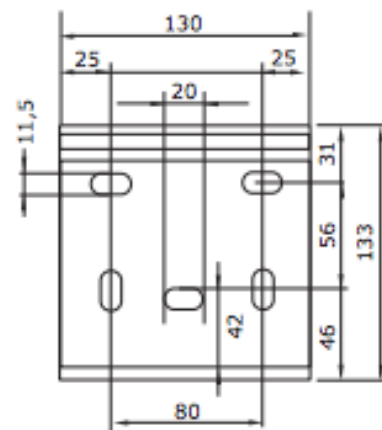
Vooraanzicht muursteun
